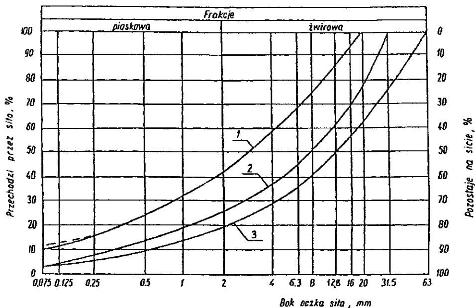
Rysunek 1. Pole dobrego uziarnienia
