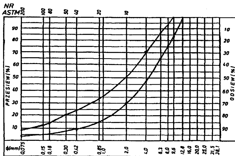
Rys. 4. Krzywe graniczne uziarnienia mieszanki mineralnej 0-16 mm do podbudowy z betonu asfaltowego dla KR 1-2
