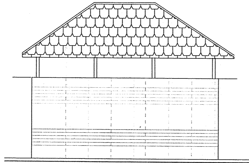
ELEWACJA BOCZNA skala 1:50
