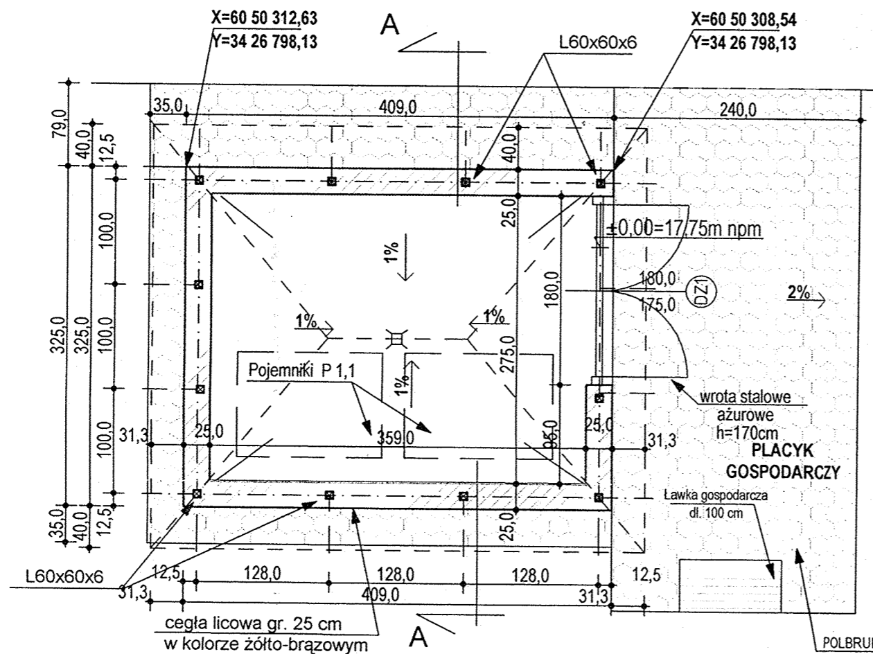
RZUT PRZYZIEMIA skala 1:50
