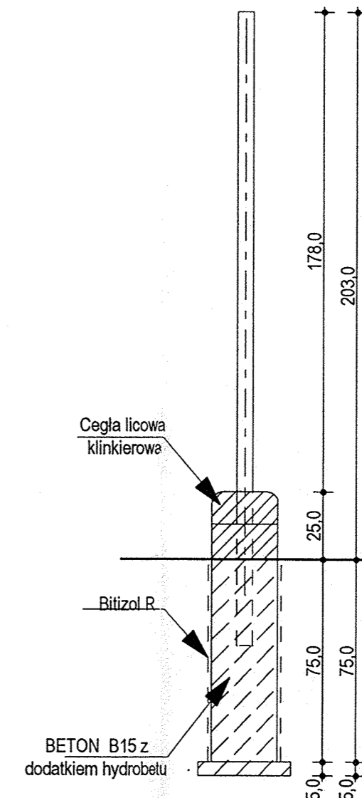
PRZEKRÓJ PIONOWY
