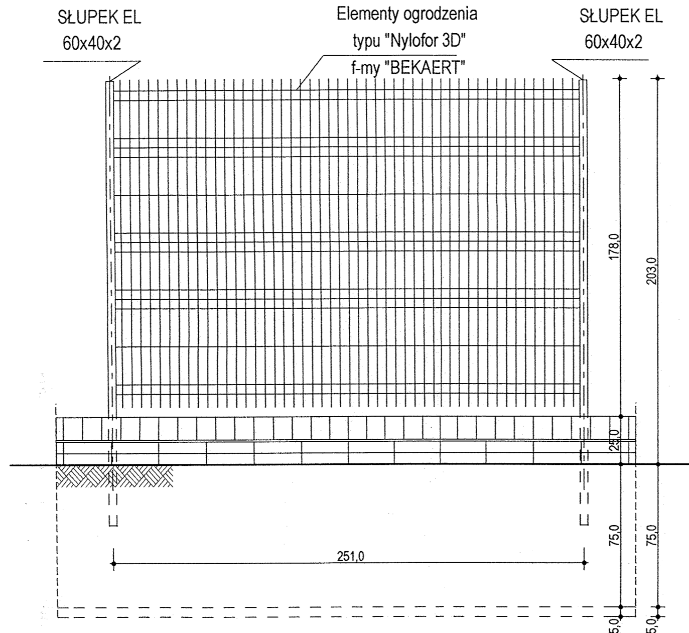
WIDOK
