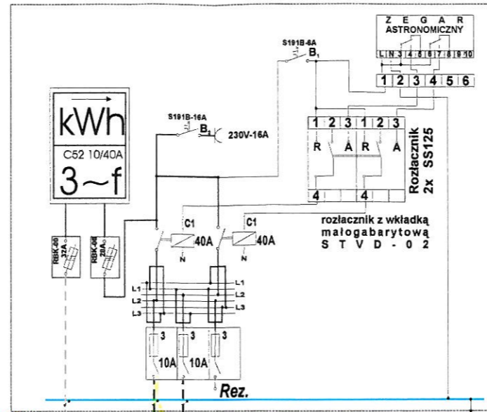
Projektowana szafka oświetleniowa
